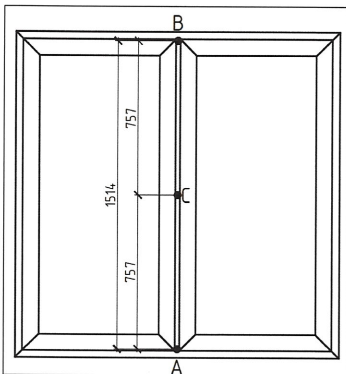
Рисунок 9 – Схемы расположения датчиков линейного перемещения при испытании образца 994-24-2-2 на сопротивление ветровой нагрузке
