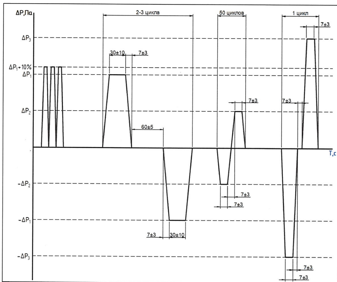
Рисунок 10 – Порядок проведения испытаний образца 994-24-2-2 на сопротивление ветровой нагрузке
