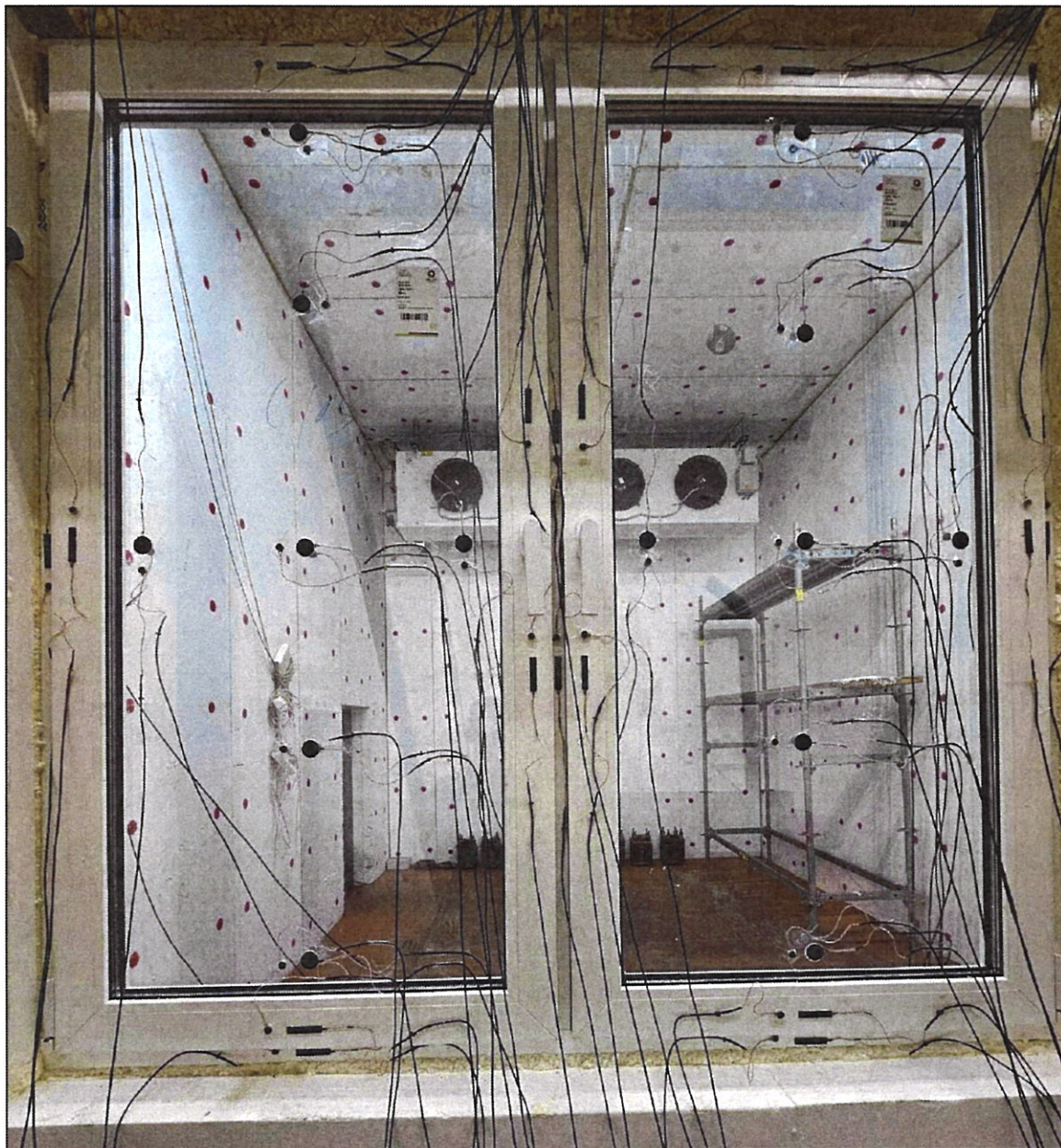
Рисунок 11– Внешний вид образца 994-24-2-1 в процессе испытаний по определению его приведенного сопротивления теплопередаче
